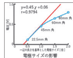
▲図4 電極面積による発生電圧の変化
