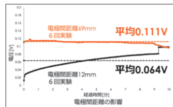
▲図3 電極間距離による発生電圧の変化
